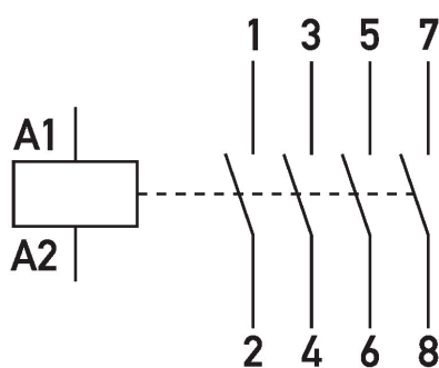
Anschlussschema HS, 230 V AC, brummarm
