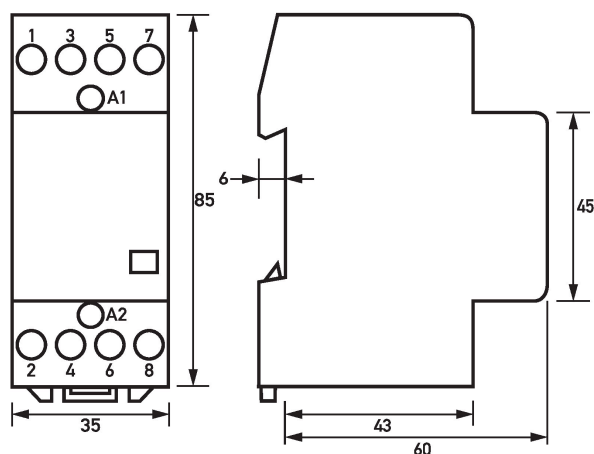
Maßzeichnung HS, 230 V AC, brummarm (Gruppenansicht)
